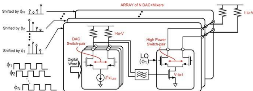
Fig. 3.28 Power Mixer Array
