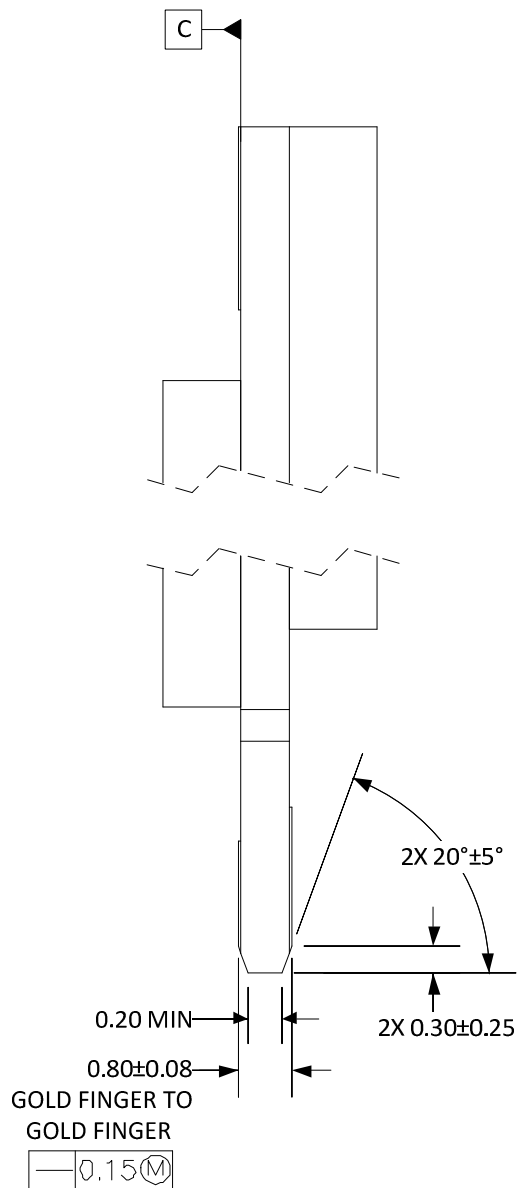
Figure 15. Card Edge Bevel
